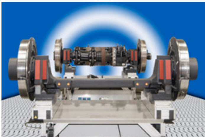
Révision des roues indépendantes sur axes latéraux
