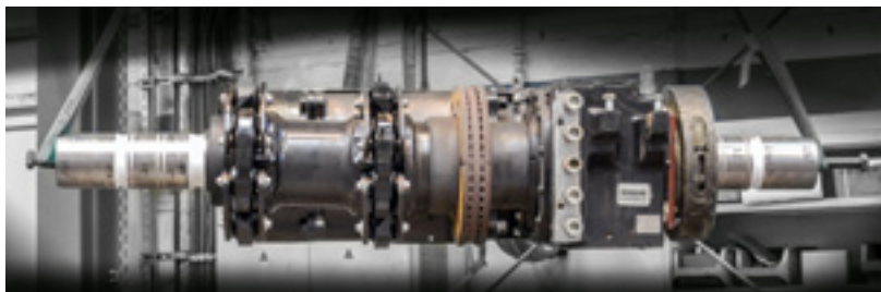
Révision des essieux montés porteur et moteur
